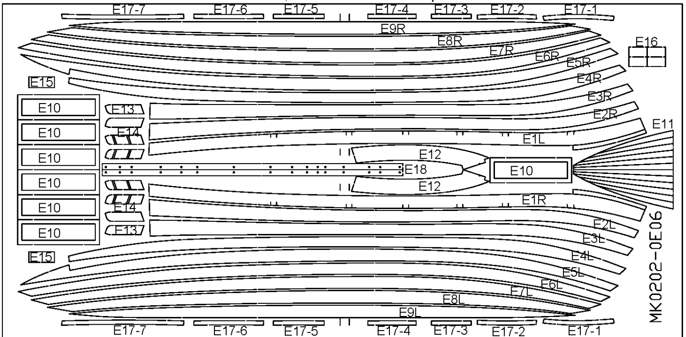
МК0202-0E06, шпон анегри 0.6 мм
