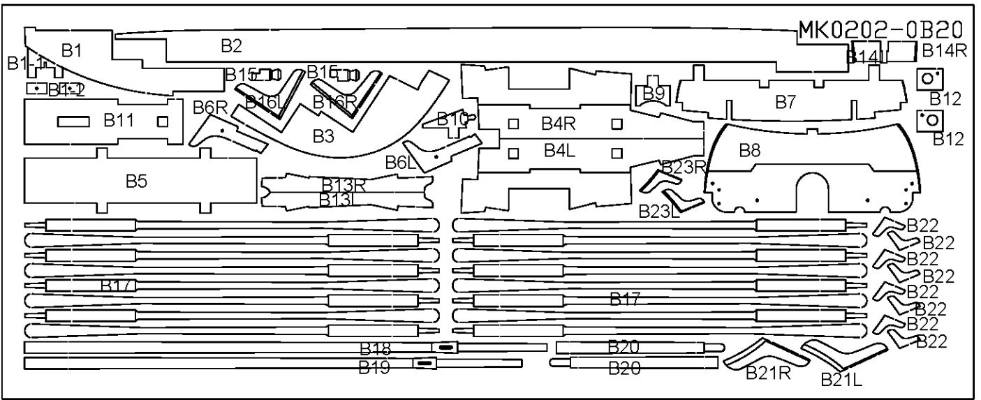
МК0202-0В20, груша 2 мм
